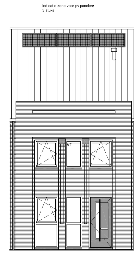
voorgevel
